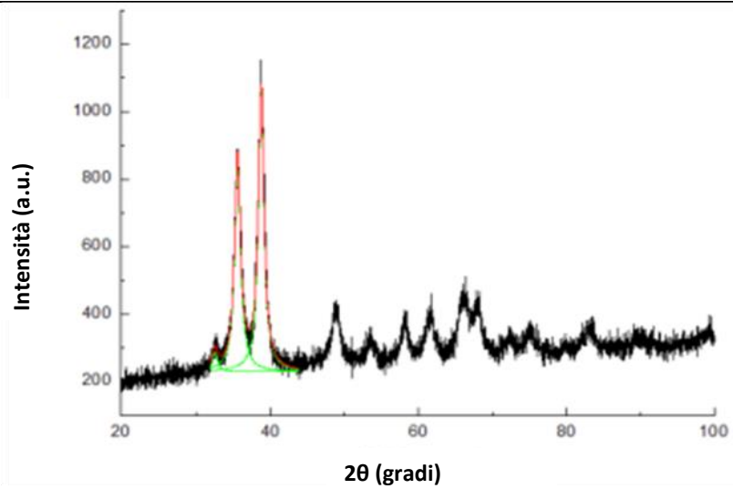
Diffrazione ai raggi X
